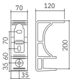
Supporto universale
