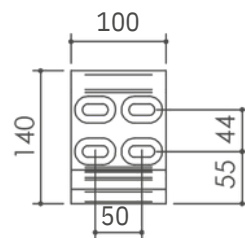
Supporto parete/soffitto
