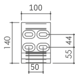
Supporto parete/soffitto
