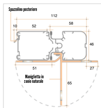
Ingombro Cassonetto e Barra maniglia.
